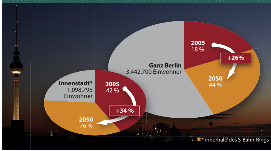
Belastendes Bioklima in der Nacht – Anteil betroffener Einwohner bis 2050 41
